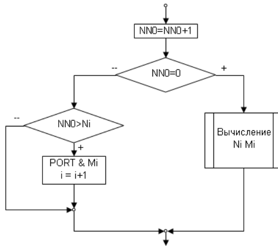
Рисунок 1. Экономичный алгоритм формирования ШИМ сигнала
