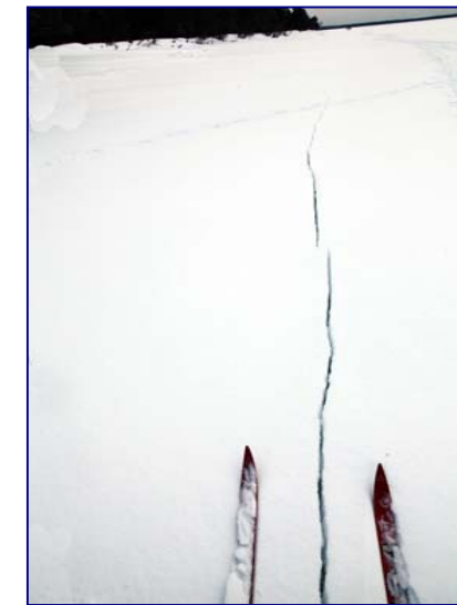
Рис. 4. Приливная трещина
